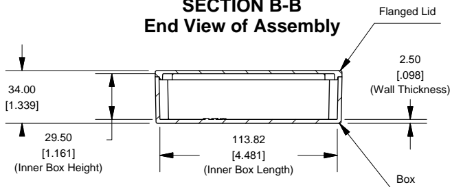
Flanged Lid
