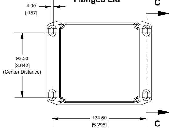
Flanged Lid
